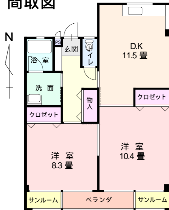
Aタイプ 2LDK 101・103・201・203号室
