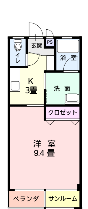
Dタイプ 1K 302・303・305・306号室
